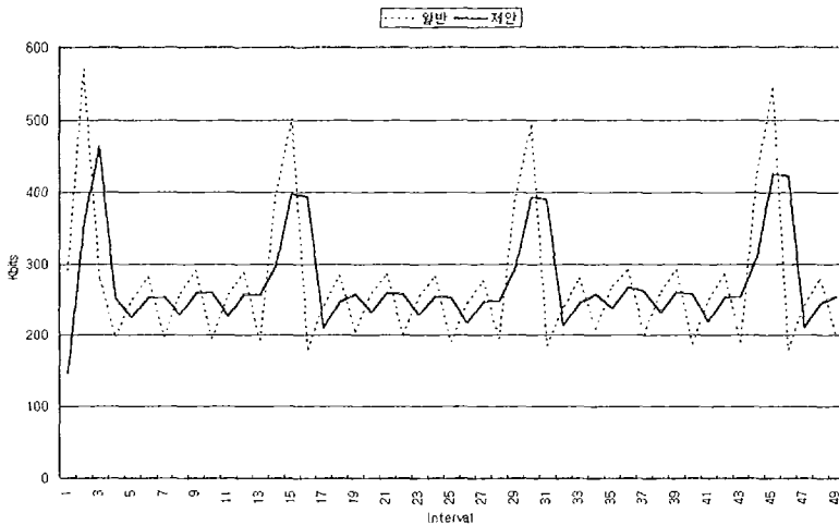
[그림 6] 다수의 입력이 임의의 시간에 전송을 개시할 경우의 출력 비교
