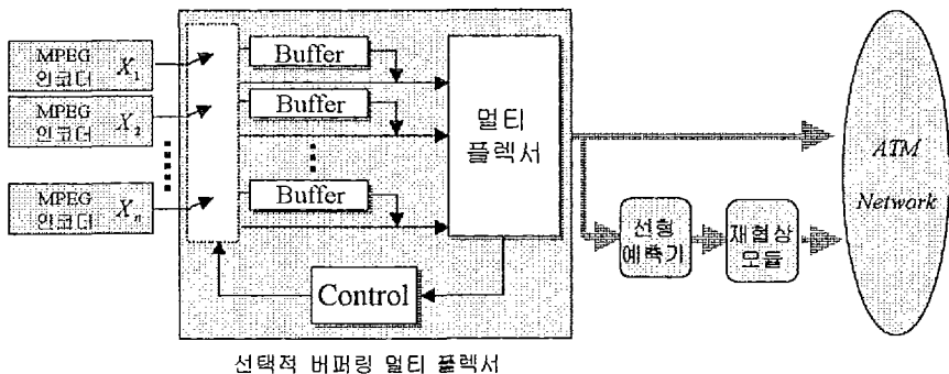
[그림 1] 선택적 버퍼링 멀티플렉서를 이용한 대역폭 재협상 모델
