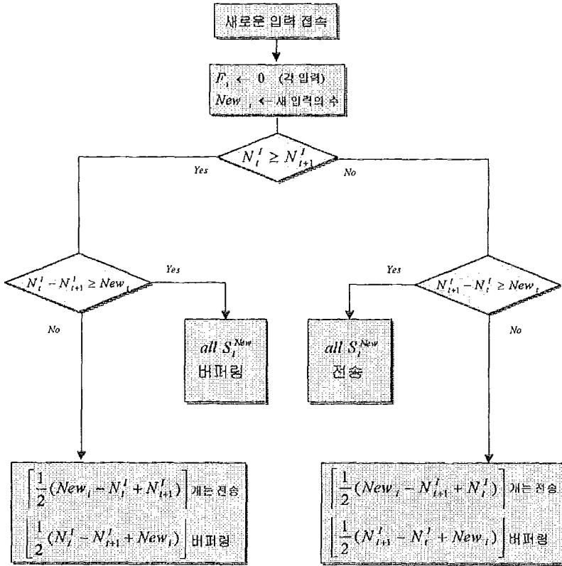
[그림 3] 멀티플렉싱 제어 알고리즘
