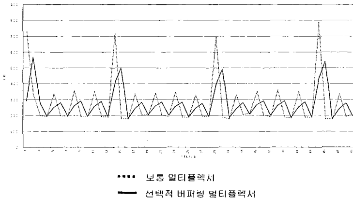
[그림 5] 동시에 다수의 입력이 전송을 개시할 경우의 출력 비교
