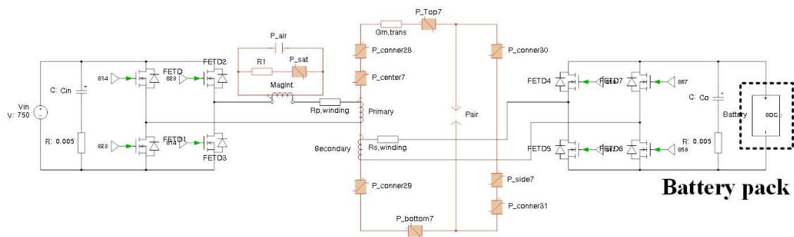
그림 3.19. 배터리 팩 충전기 에너지 효율 시뮬레이션을 위한 PLECS 회로.
