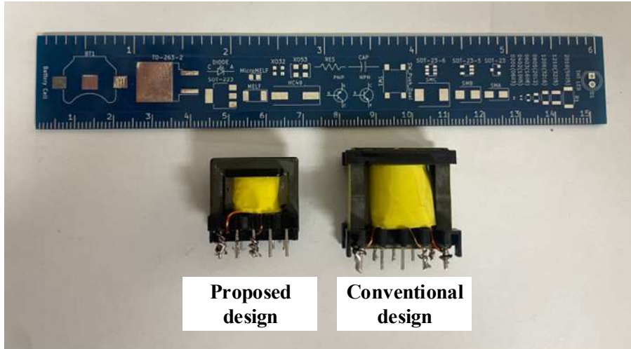
그림 4.1. 설계된 변압기 테스트 샘플.
