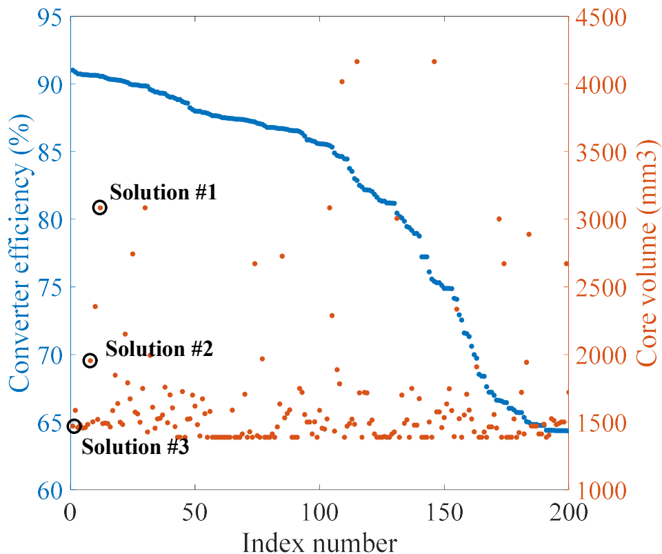
그림 3.11. 배터리 균등화 회로 파레토 전선 전력 효율 시뮬레이션 결과.
