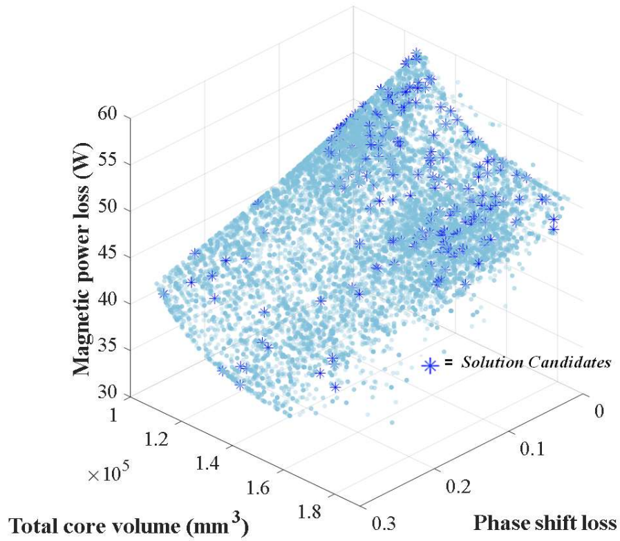
그림 3.16 계산된 배터리 팩 충전장치 Pareto front.
