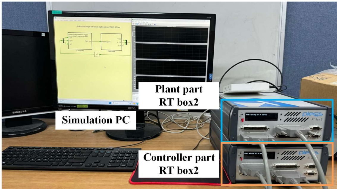
그림 4.5. 배터리 팩 충전장치 HILS 실험 구성.
