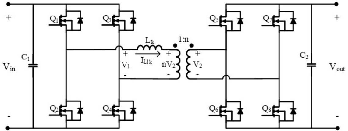
그림 3.13. 배터리 팩 충전기 컨버터 구조.
