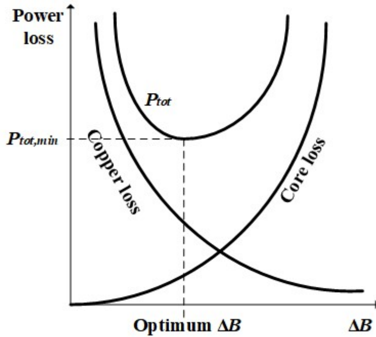
그림 2.3. 최대 자속밀도와 변압기 총 손실 관계.
