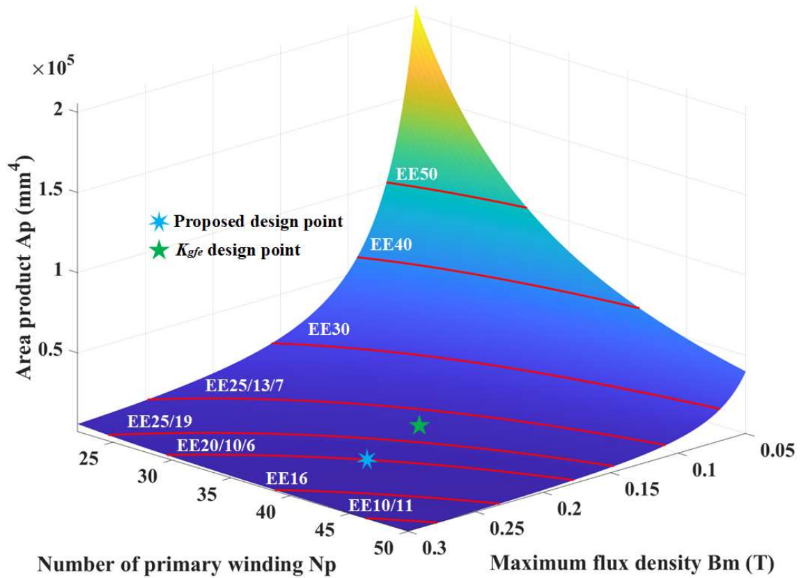
그림 3.12. N_p , B_m 에 대한 변압기 코어 선정 A_p 포인트 ( N=5 ).
