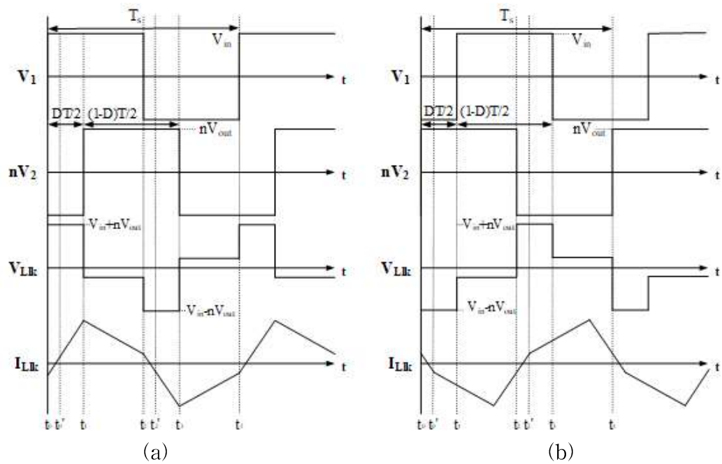
그림 3.14. 배터리 팩 충전기 컨버터 파형: (a) 벡 모드( D > 0 ); (b) 부스트 모드( D < 0 ).
