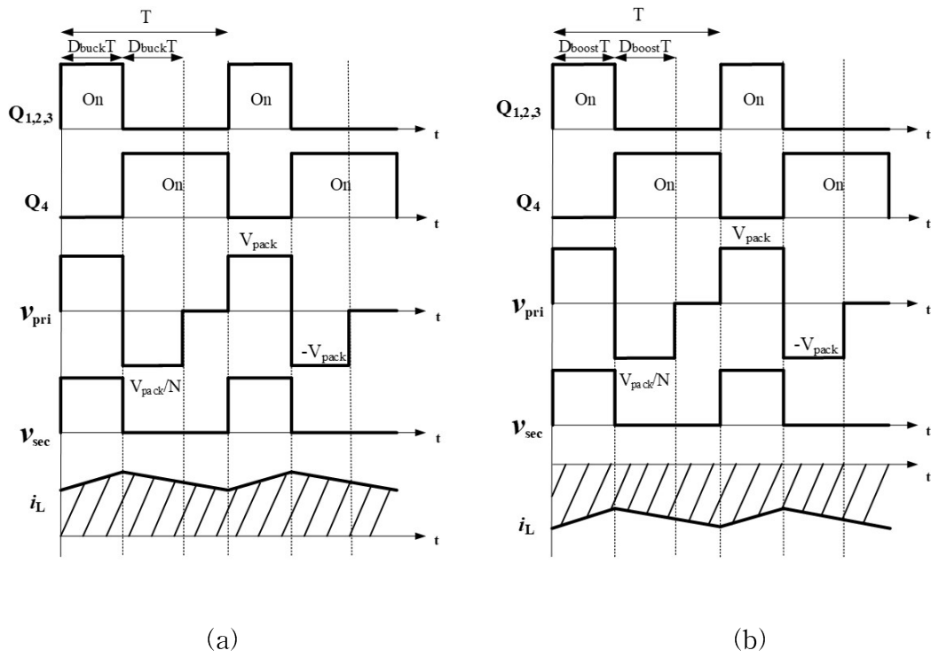
그림 3.5. 배터리 균등화 회로 컨버터 동작 파형: (a) 벙 모드; (b) 부스트 모드. Fig. 3.5. Battery equalizer converter operation waveform: (a) buck mode; (b) boost mode.
