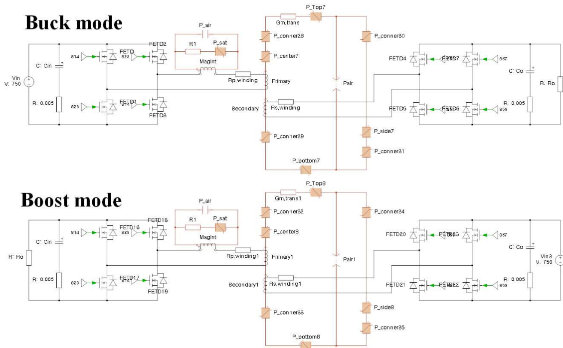
그림 3.18. 배터리 팩 충전기 전력 효율 시뮬레이션을 위한 PLECS 회로.
