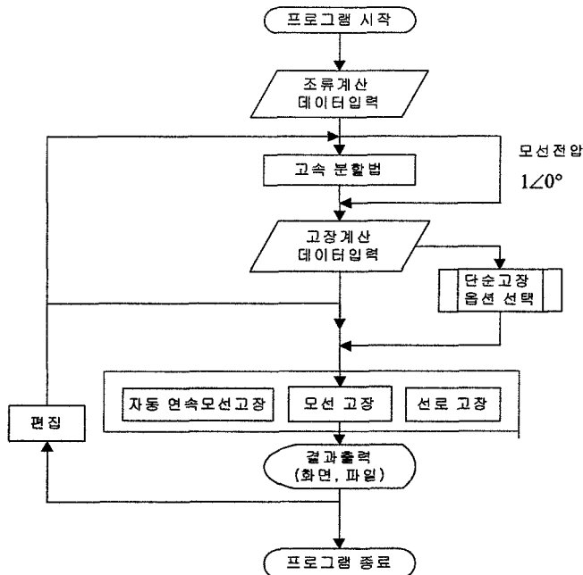
그림 6. 프로그램의 수행과정
