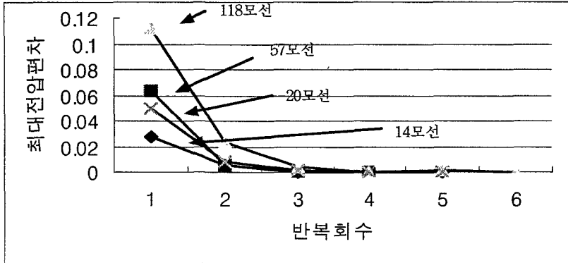
그림 7. 샘플계통의 수렴특성
