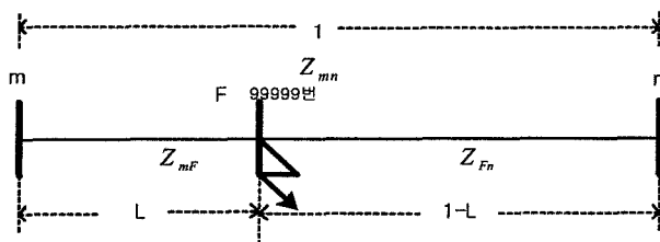
그림 1. 선로고장의 예
